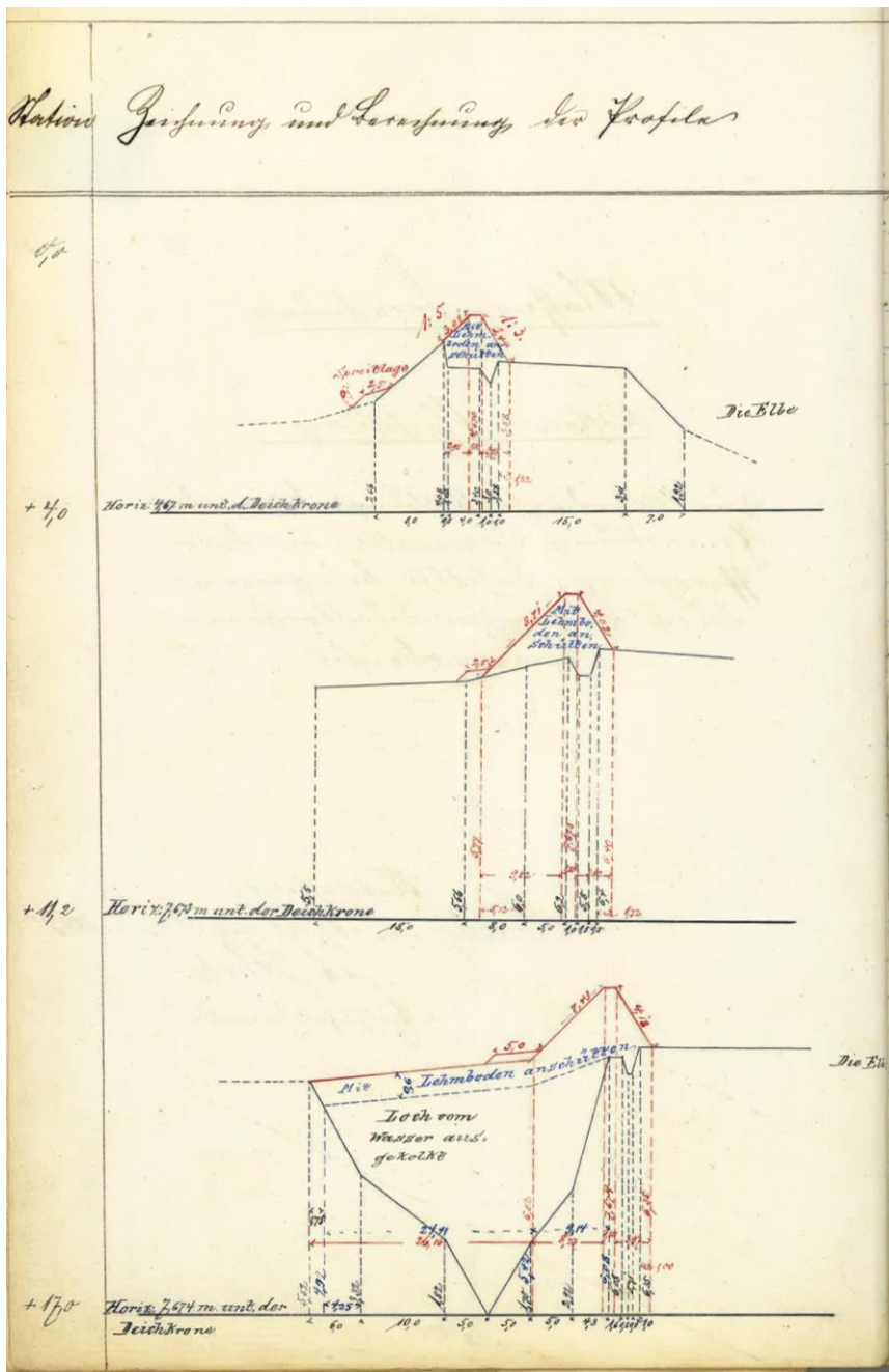
Zeichnungen und Berechnungen der Profile
